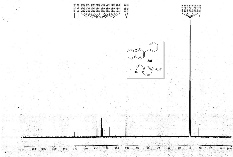
^{13}\text{C-NMR} of 3af
